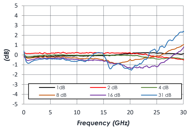
Attenuation Error
