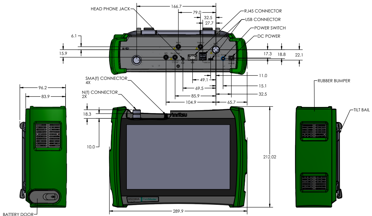
MS2080A
