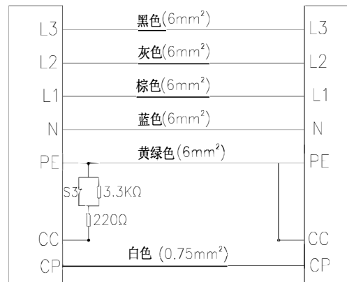
国标车辆端接线图
