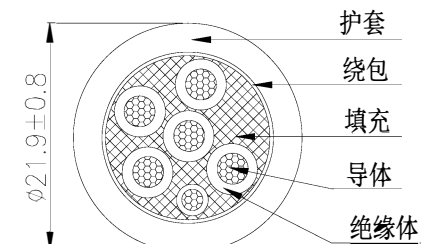
SEC A-A
