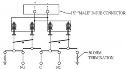
15 Pin D-Sub
