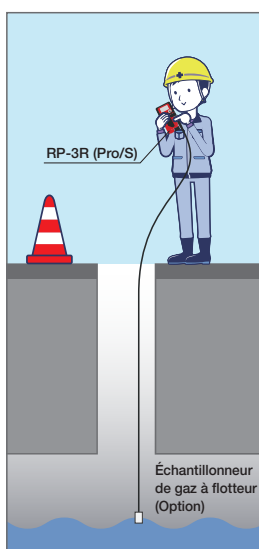
Échantillonneur de gaz à flotteur (Option)
