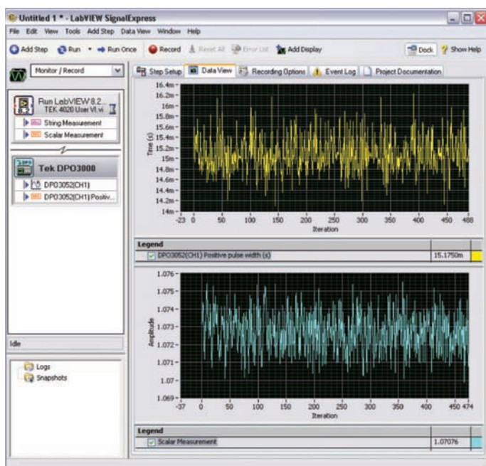
Acquisition des données provenant des modèles DMM4020 et DP03052 de Tektronix par Signal Express.
