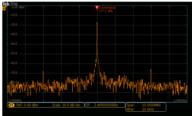
MDO3000 - Affichage du domaine fréquentiel.
