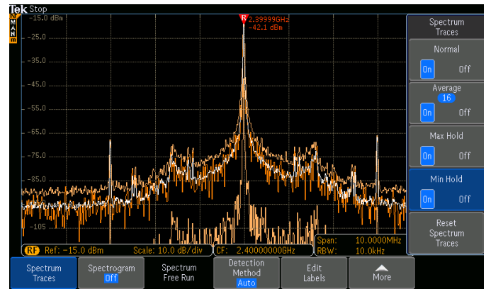
Traces de spectre Normal, Average, Max Hold et Min Hold
