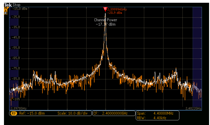
Mesure automatique de puissance
