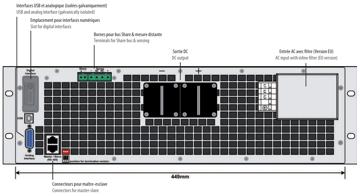
Vue arrière du modèle de base
