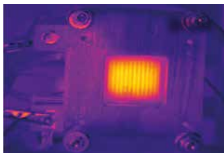
Chargement d'une pile à combustible à membrane
