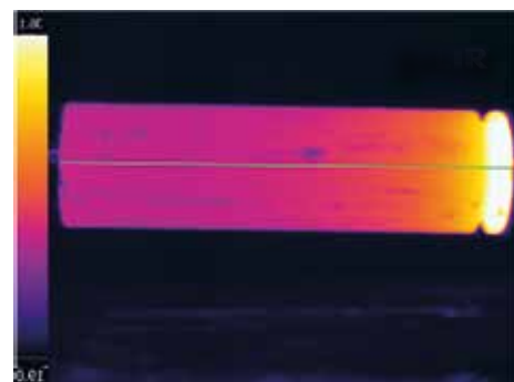
Gradient thermique d'une batterie 18650 en décharge
