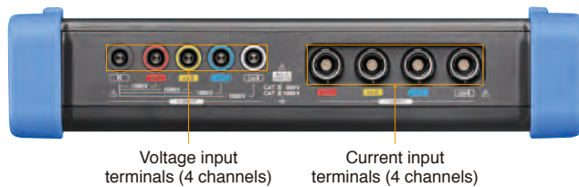
PQ3100 top
